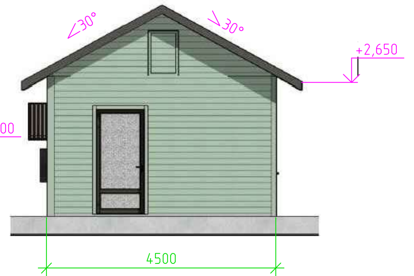
Тыльный фасад
